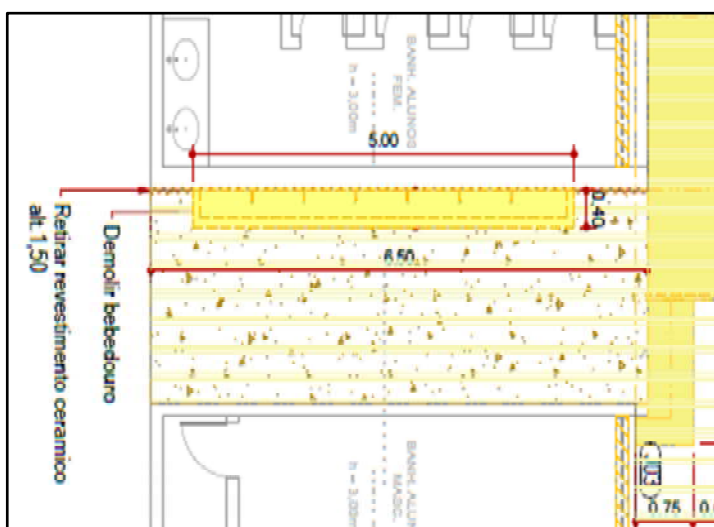
Figura 2 – Recorte da folha 1 do projeto, onde a demolição do bebedouro.
