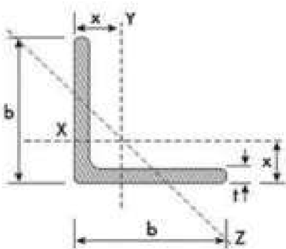
Imagem 37 – Parâmetros de identificação do perfil cantoneira de abas iguais.
