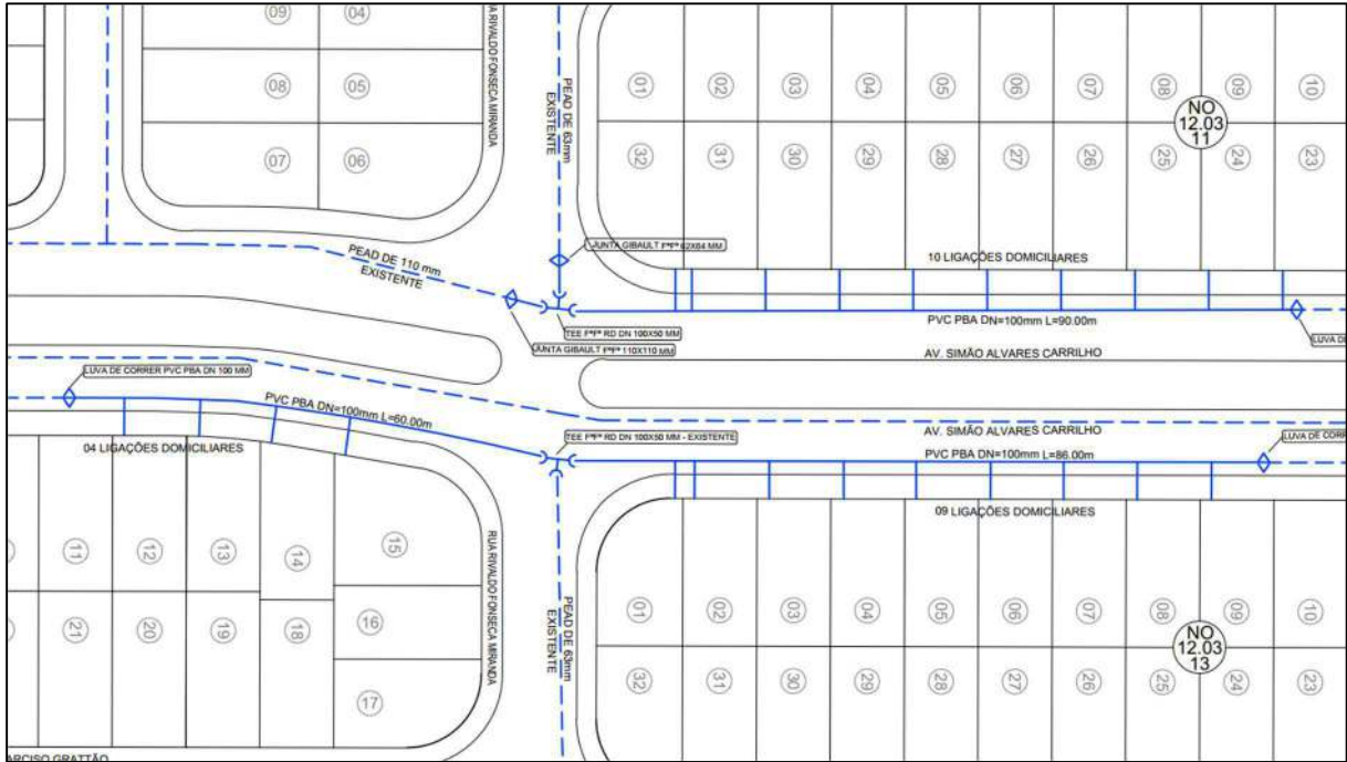
Figura 3 - Trecho Já Substituído na Av. Simão Alvares Carrilho, representado pela a linha azul contínua, trechos existentes representados pelas linhas azuis pontilhadas.
